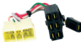
Mini Excavator John Deere/Kubota
